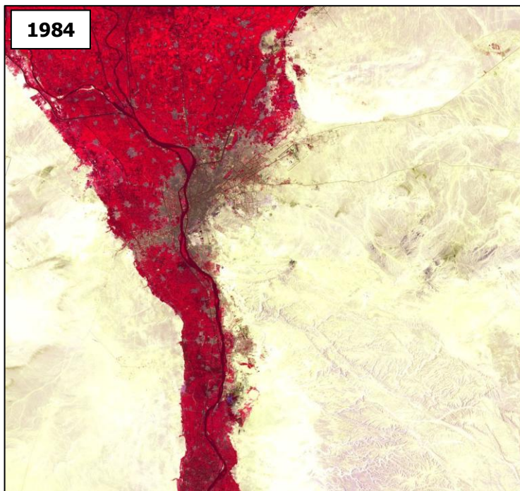
Image Landsat 4-5 (TM/Fausses couleurs), 3 août 1984, U.S. Geological Survey.
