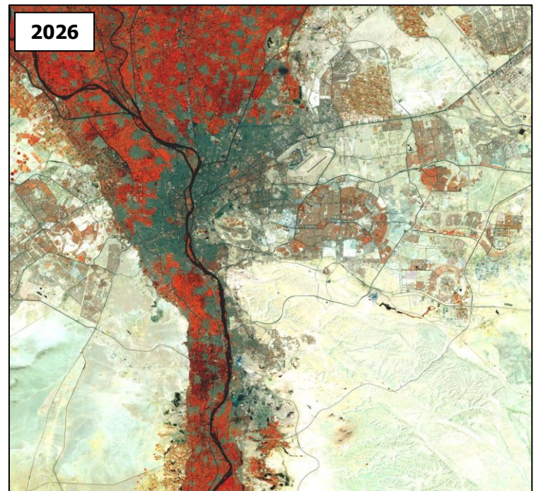
Image Landsat 8 (OLI/Fausses couleurs), 25 avril 2026, U.S. Geological Survey.
